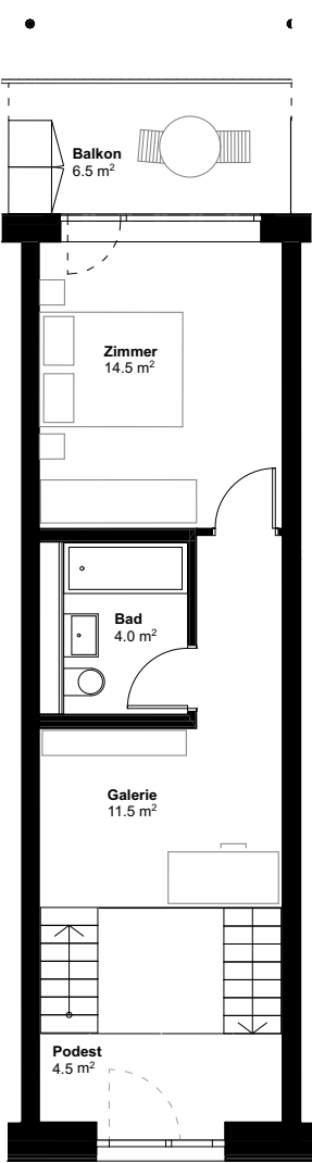
1.OG
